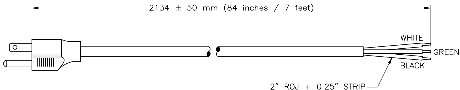
NEMA 5-15P
