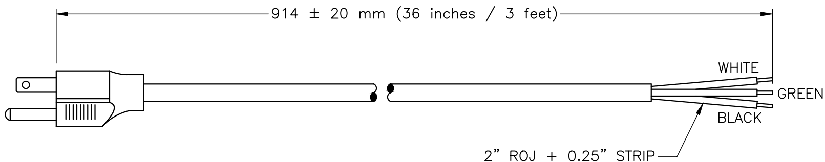
NEMA 5-15P
