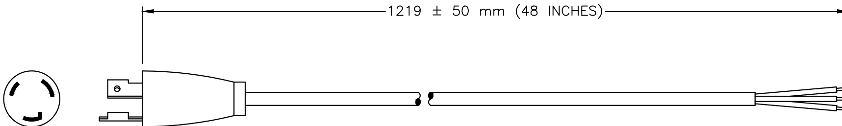
NEMA L6-20P
