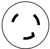
NEMA L6-30P
