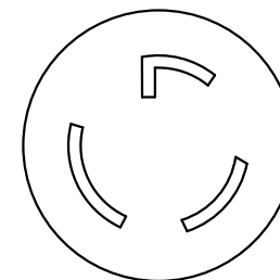
NEMA L5-30R (CONNECTOR SIDE)
