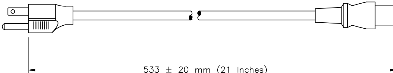
IEC 60320 C-15
