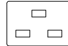
IEC 60320 C15 (CONNECTOR SIDE)
