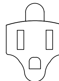
NEMA 5-15R (CONNECTOR SIDE)
